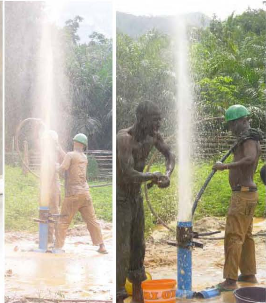
Dazu eine Tiefbohrung, die aus 72 m Wasser fördert
